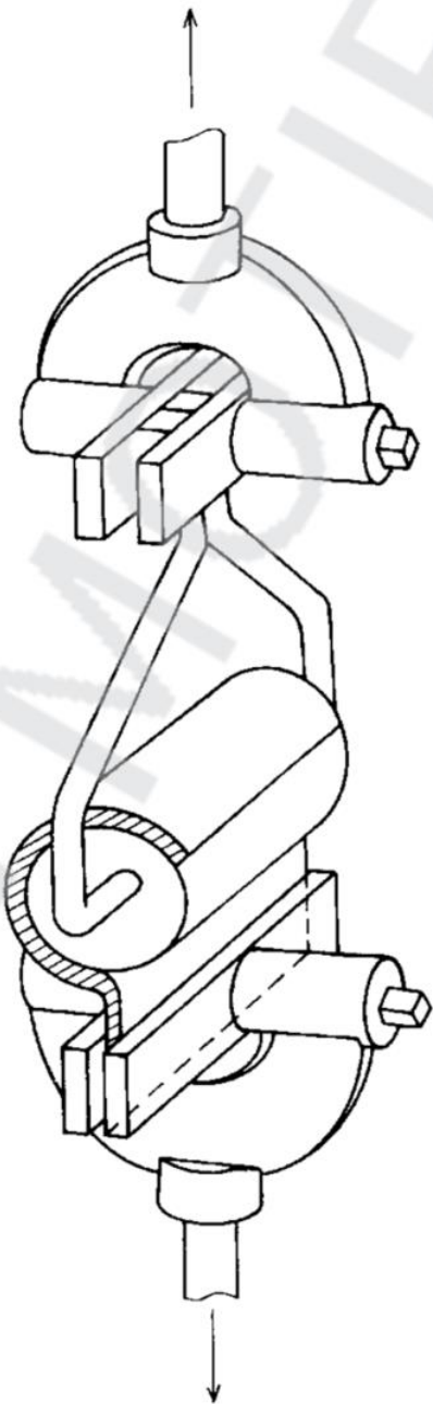
그림 A.2 — 박리 강도 시험 장치(보기)
