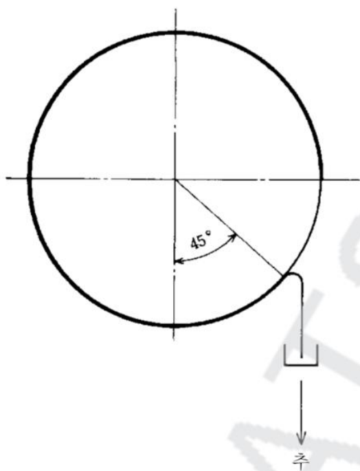
그림 A.1 — 박리 속도 시험(보기)
