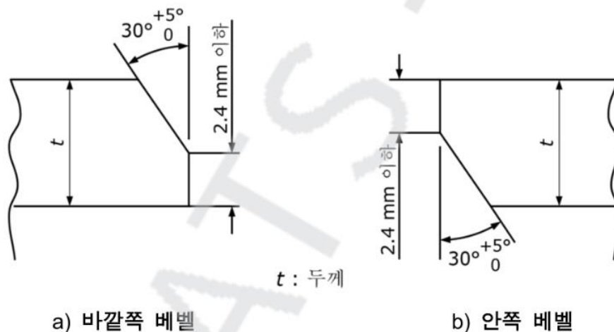
그림 1 — 베벨 엔드의 모양
