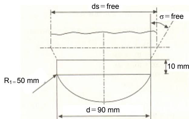
그림 2 - 추의 모양 및 치수
