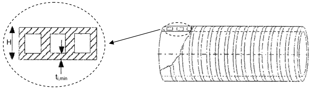
그림 1 - 이중벽관
