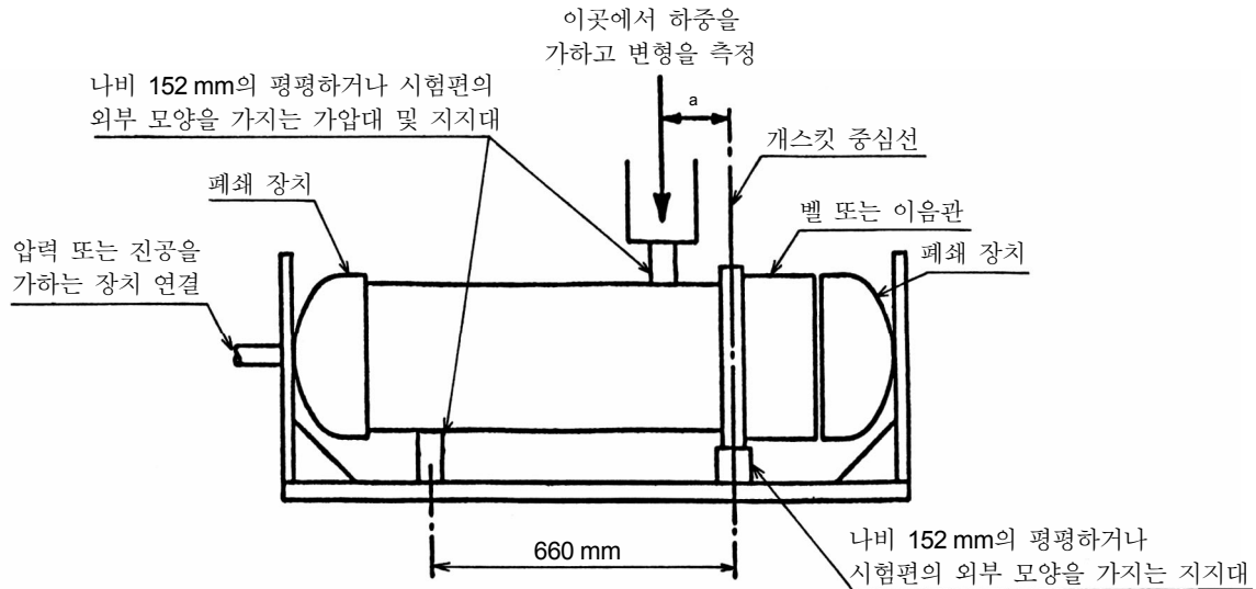
그림 3 - 시험편
