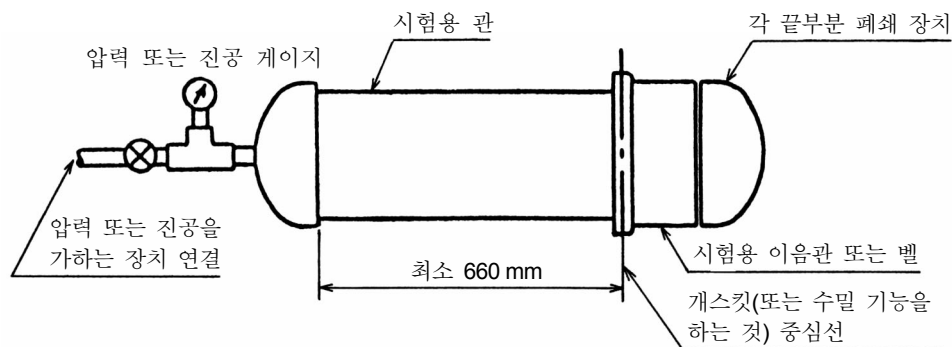
그림 3 - 시험편
