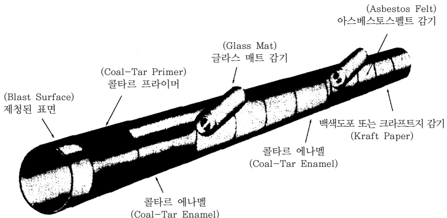
그림 1.31 도복장(예)
