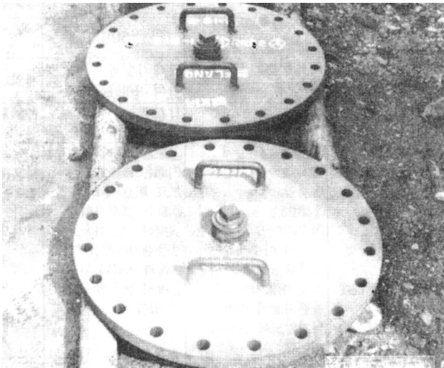
사진 : 맨홀겸용 맹플랜지
