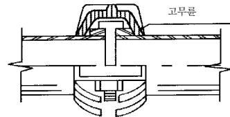
그림 1.8 빅토리형 신축이음
