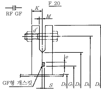
RF-GF(홈 형)
