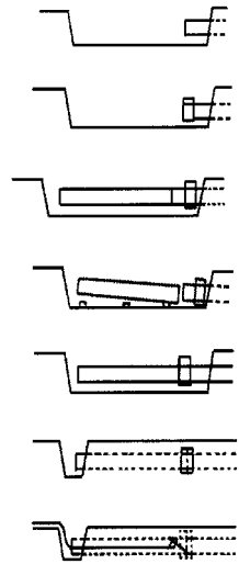
그림 3.22 급속매설공법의 개요도
