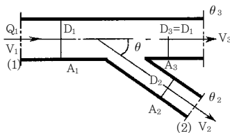
그림 2.12 분기관
