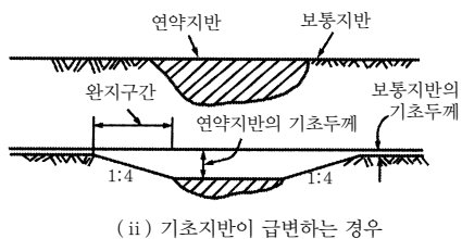
그림 3.4 연약지반에서의 기초
