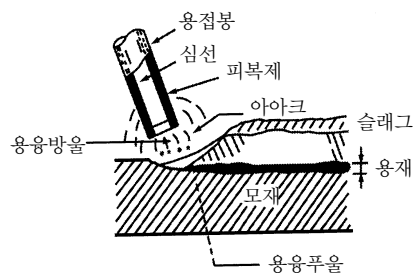
그림 3.6 피복아아크용접의 상황
