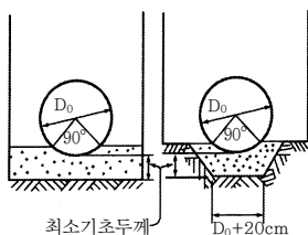
그림 3.3 보통지반의 경우
