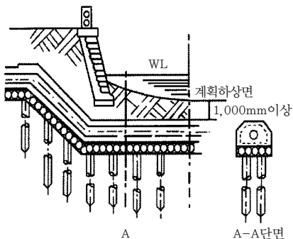
그림 3.19 하저횡단의 예
