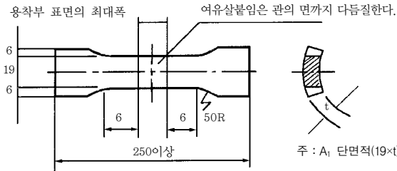
그림 1.32 2호 시험편
