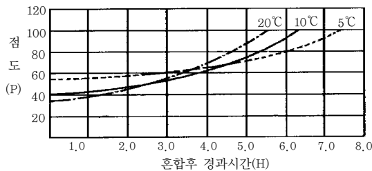
해설 그림 2 기온이 점도 변화에 미치는 영향의 보기
