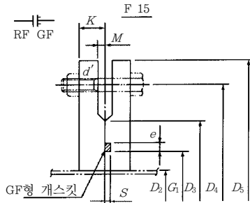
RF-GF(홈 형)
