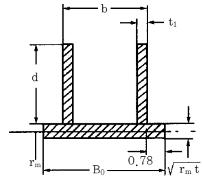
그림 2.30 링의 단면
