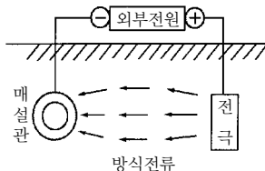
그림 1.33 외부전원법의 예
