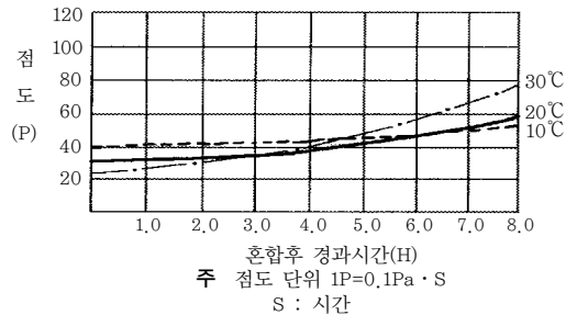
해설 그림 1 기온이 점도 변화에 미치는 영향의 보기
