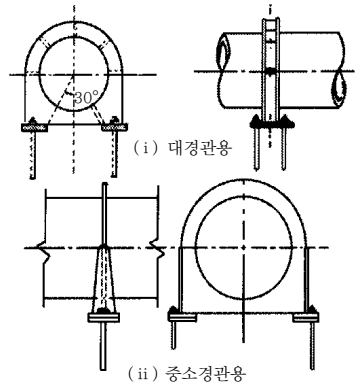
그림 2.31 링 씨포트의 설치형식
