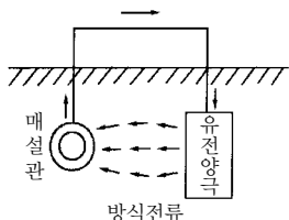
그림 1.32 유전양극법의 예
