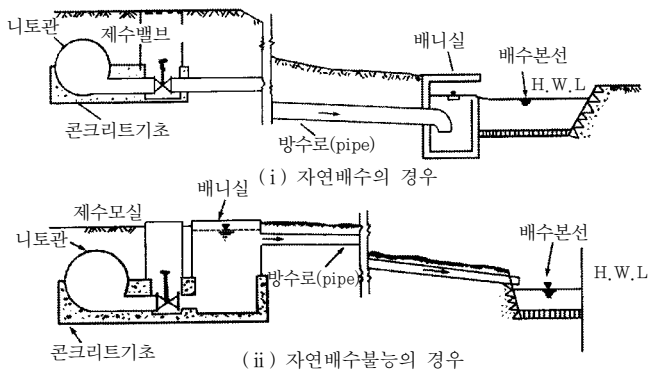
그림 1.13 배이시설의 예
