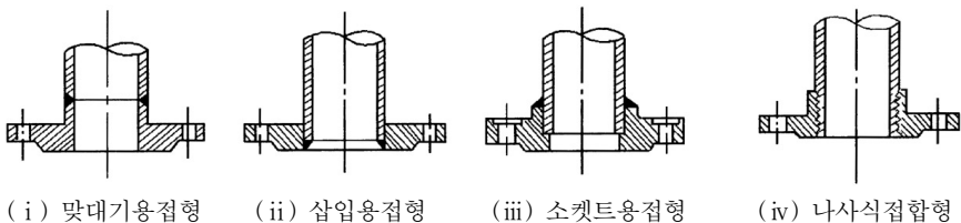
그림 1.4 접합방법별 플랜지 형상
