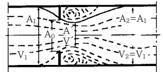
그림 2.8 관내 오리피스
