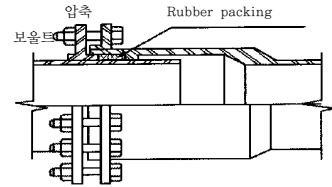
그림 1.7 텔레스코픽 신축이음
