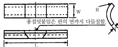
그림 1.35 판에 대한 표면굽힘 및 뒷면굽힘 시험편
