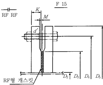
RF-RF(대평면 자리)
