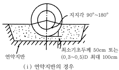
그림 3.4 연약지반에서의 기초
