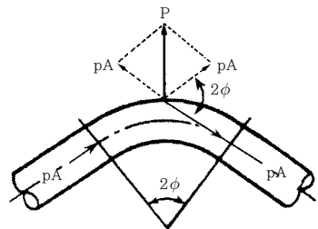
그림 2.25 수압의 불평형력
