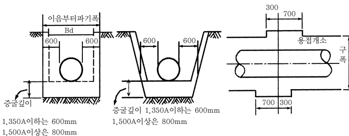
그림 3.1 강관 현장 용접접합부 터파기표준(단위mm)
