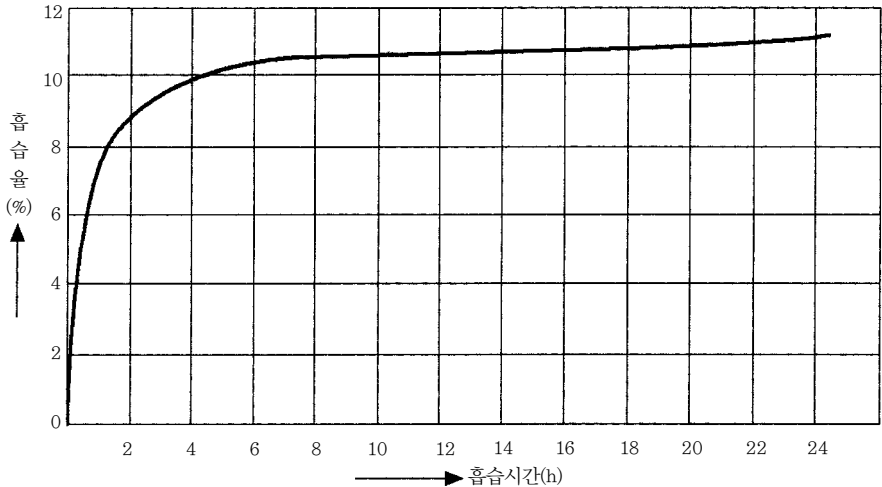
그림 1.30 건조(*) 헤시언 클로스의 흡습곡선
