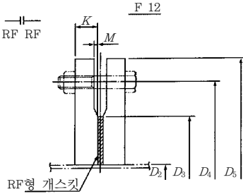
RF-RF(대평면 자리)
