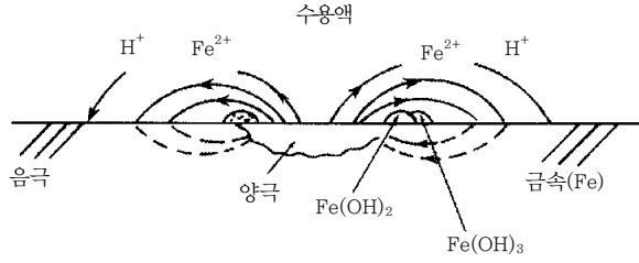
그림 1.17 매설관 부식의 전기화학적 기구
