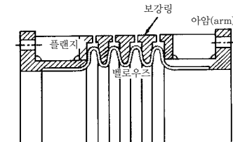
그림 1.9 벨로우즈형 신축이음
