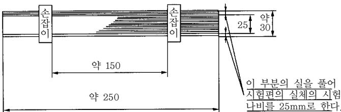
그림 2 시험편을 취하는 방법
