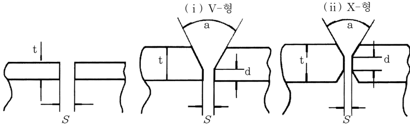
그림 1.1 플레인 엔드 접합
