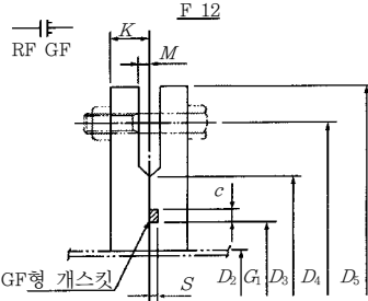
RF-GF(홈 형)
