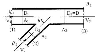
그림 2.12 합류관
