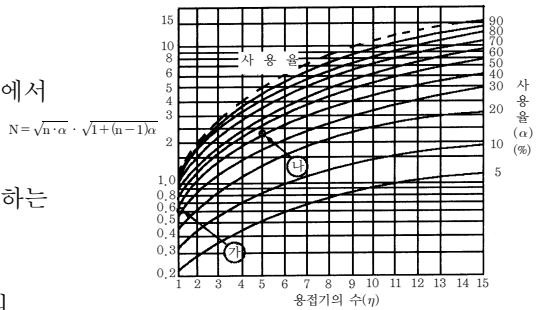
그림 3.8 전원용량의 산정용곡선
