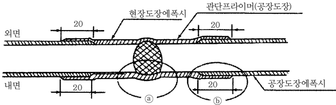
④부 상세도
