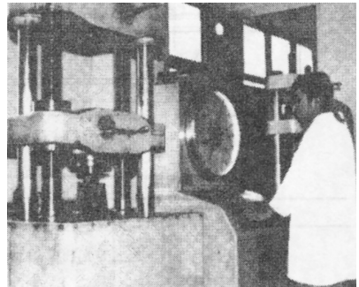
사진 : 형틀굽힘 시험 광경
