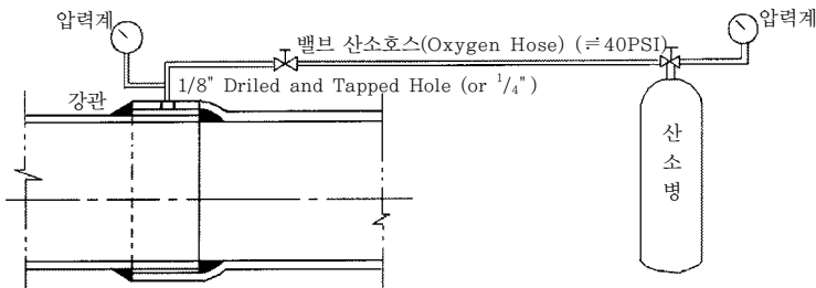
그림 3.17 벨엔드 접합부의 누설시험방법
