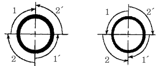
그림 3.9 현장용접 진행 순서
