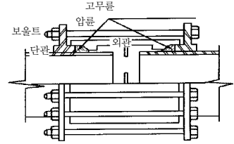
그림 1.6 드레서형 신축이음
