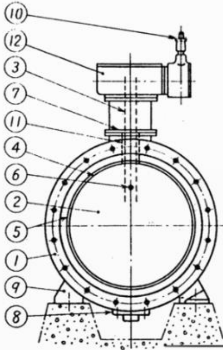
수도용 버터플라이 밸브(수직형)
