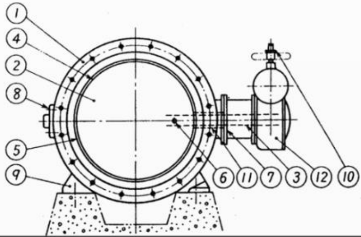
수도용 버터플라이 밸브(수평형)
