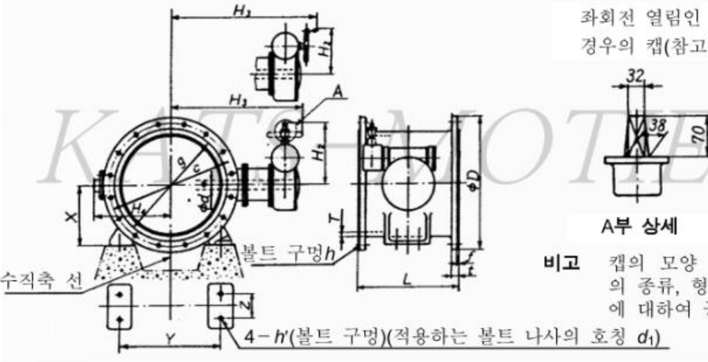
수도용 버터플라이 밸브(수평형)
