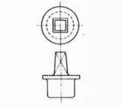
그림 1 — 캡의 모양
