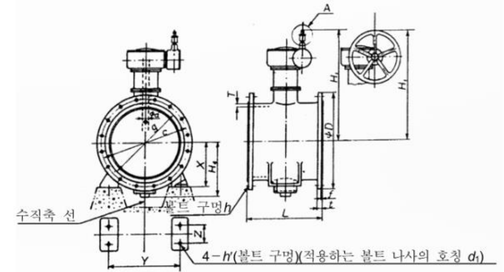
수도용 버터플라이 밸브(수직형)
