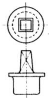
그림 1 — 캡의 모양
