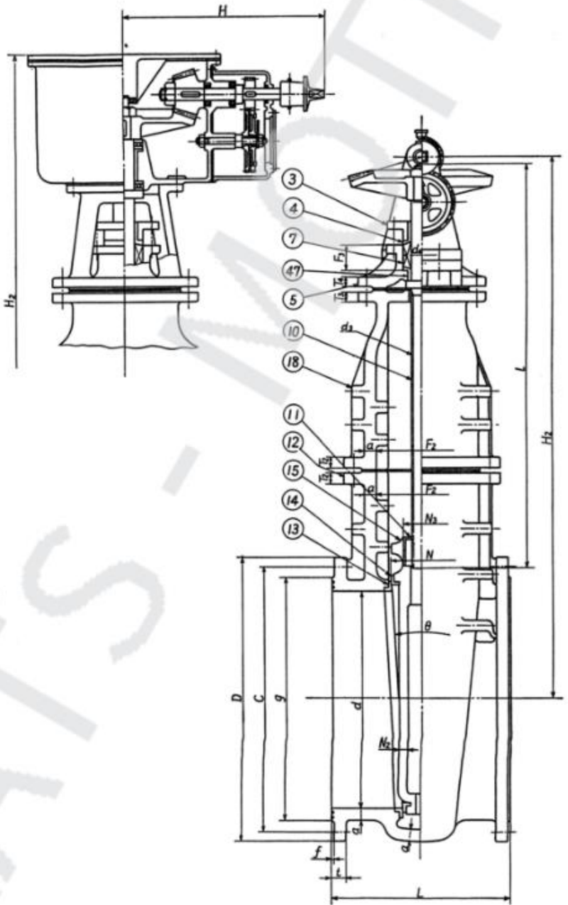
그림 5 — (호칭 지름 400~1 500) (각부의 치수 및 재료는 표 5에 따른다.)
